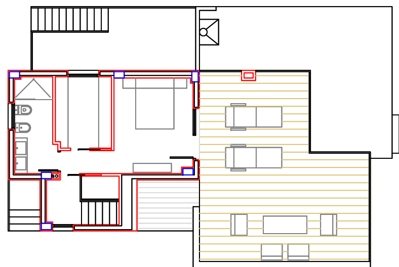
PLANTA PISO
