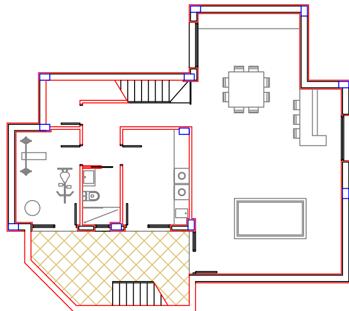
PLANTA SEMISOTANO
