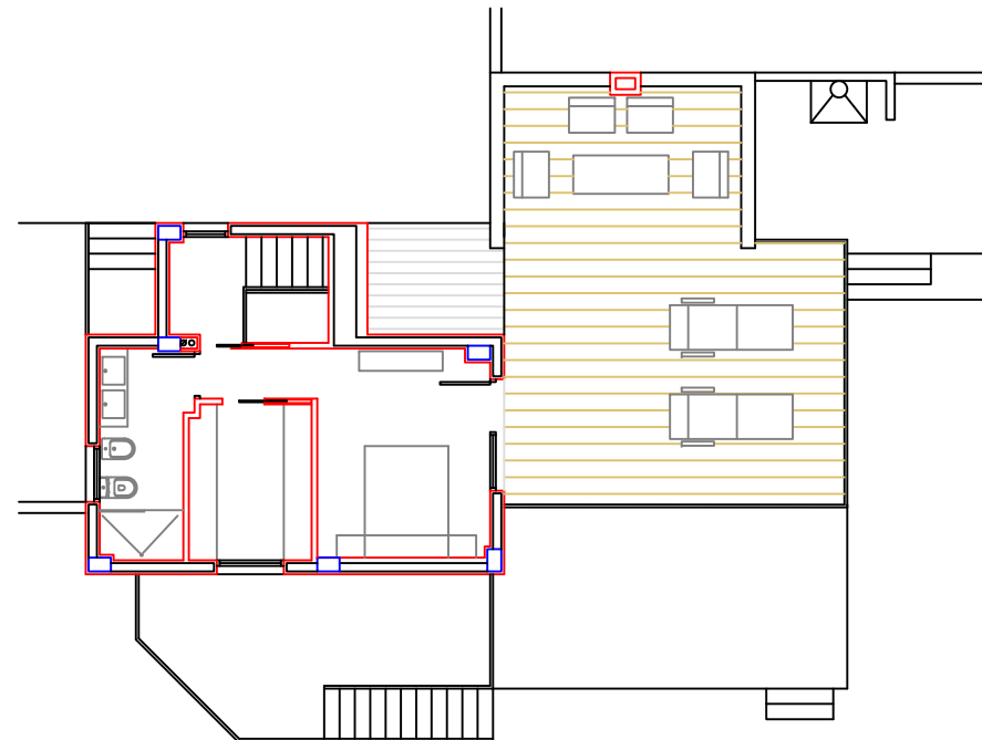
PLANTA PISO
